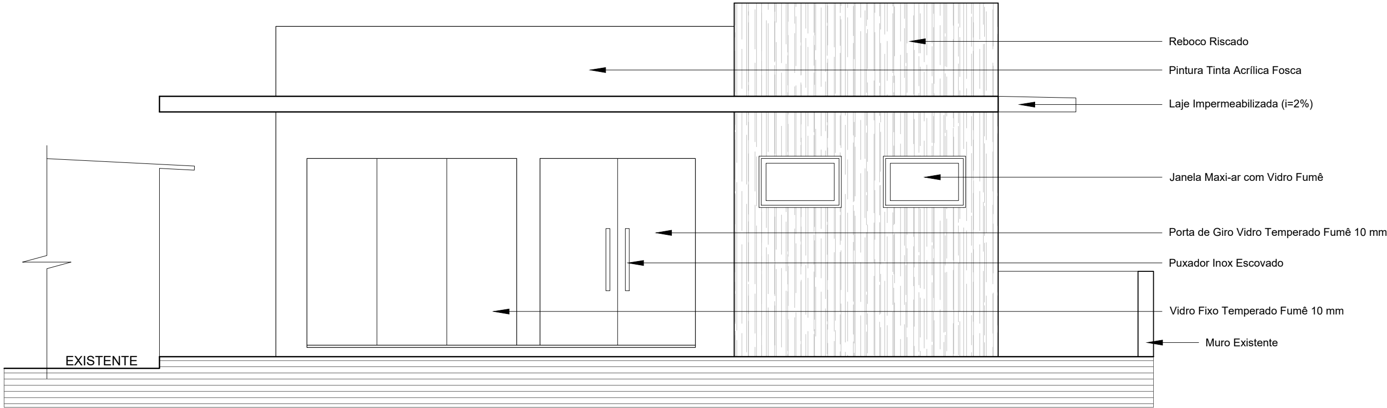
FACHADA LESTE ESC.:1/50
