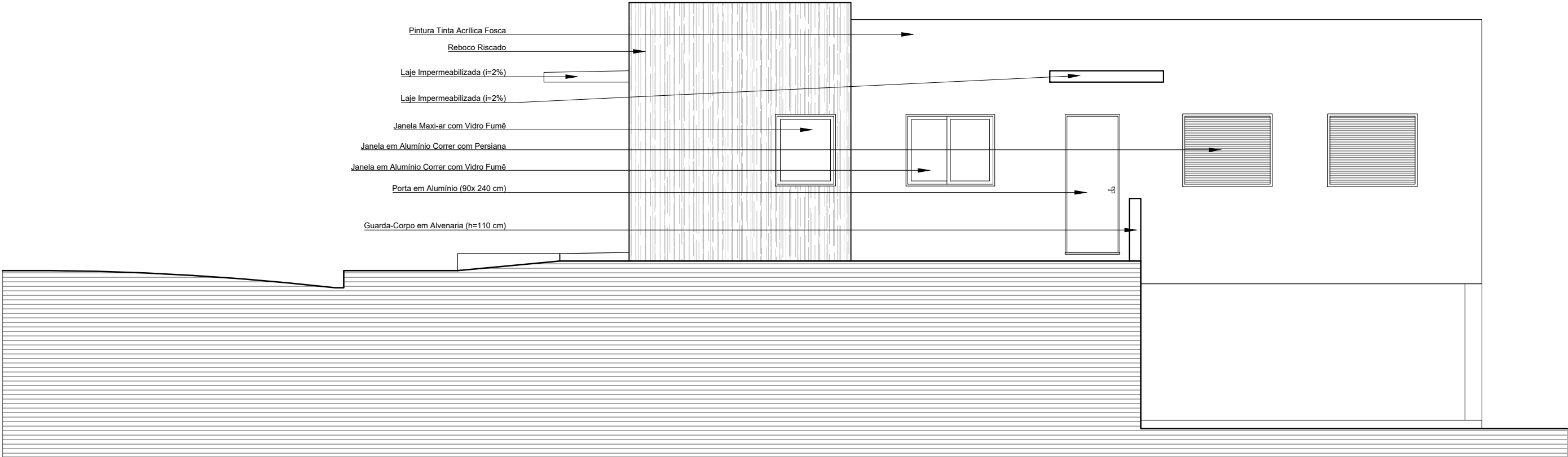
FACHADA NORTE ESC.: 1/75
