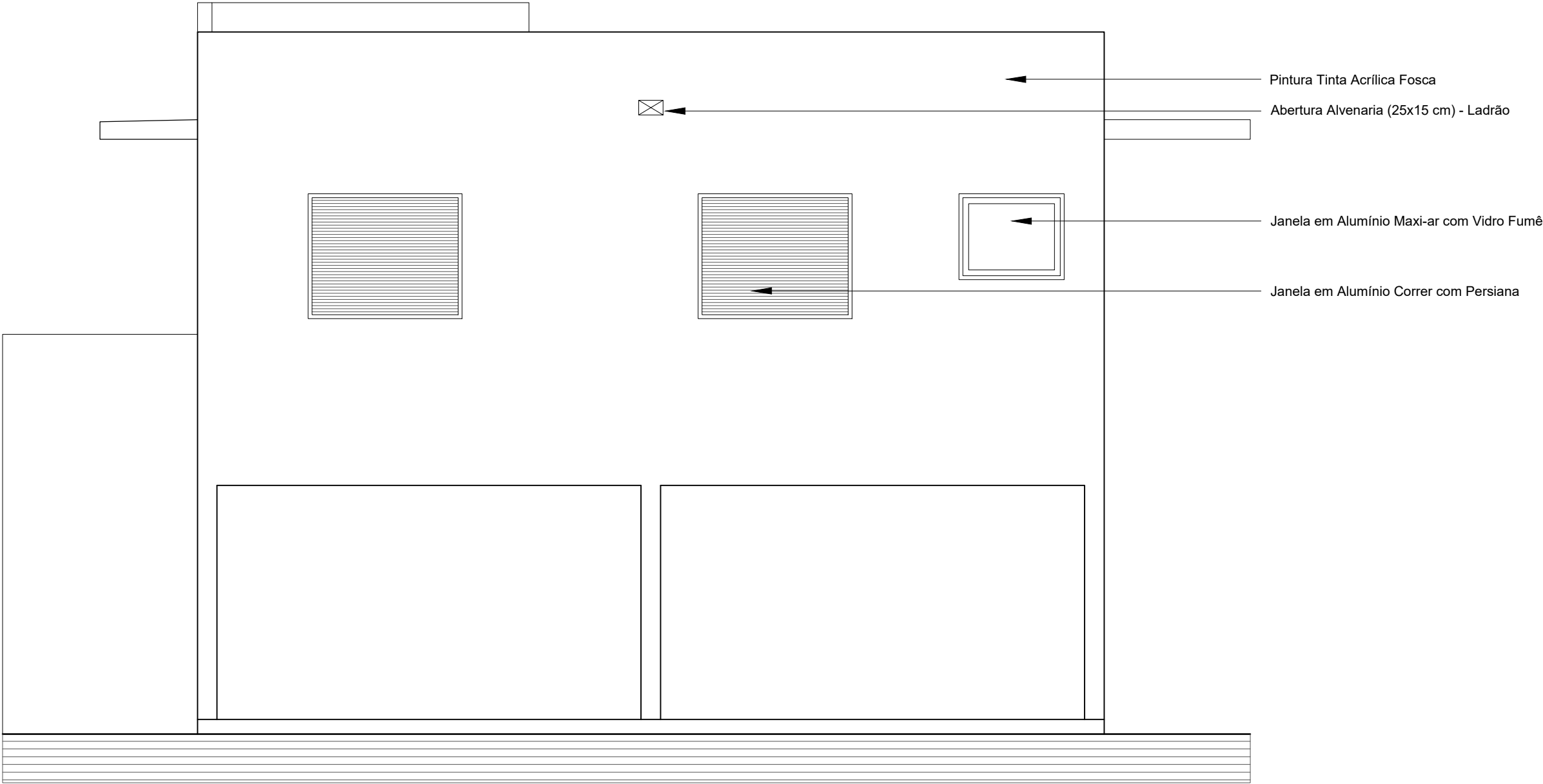
FACHADA OESTE ESC.:1/50
