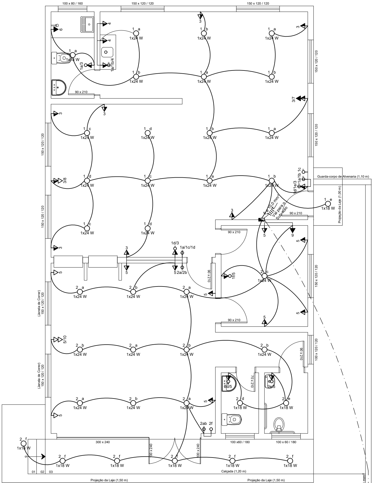
PLANTA BAIXA - TÉRREO (ELÉTRICO) ESC.: 1/75
