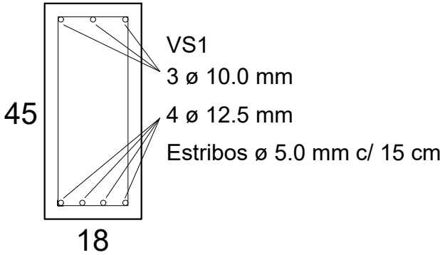
DETALHAMENTO VS - SUB-SOLO
