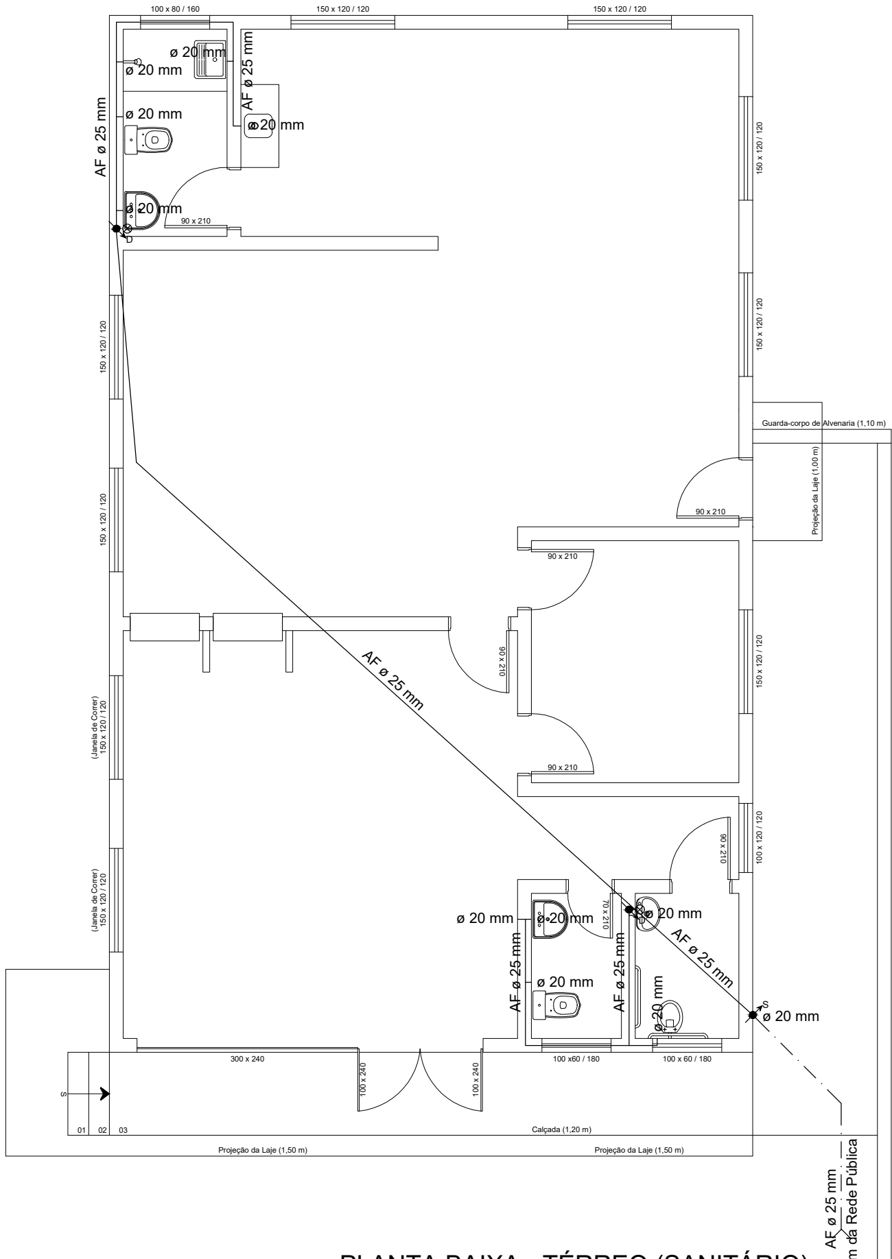
PLANTA BAIXA - TÉRREO (SANITÁRIO) ESC.: 1/75
