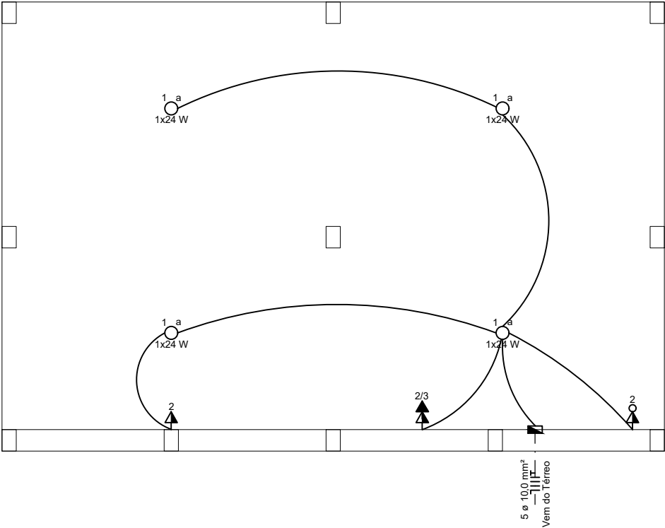
PLANTA BAIXA - SUB-SOLO (ELÉTRICO) ESC.: 1/75
