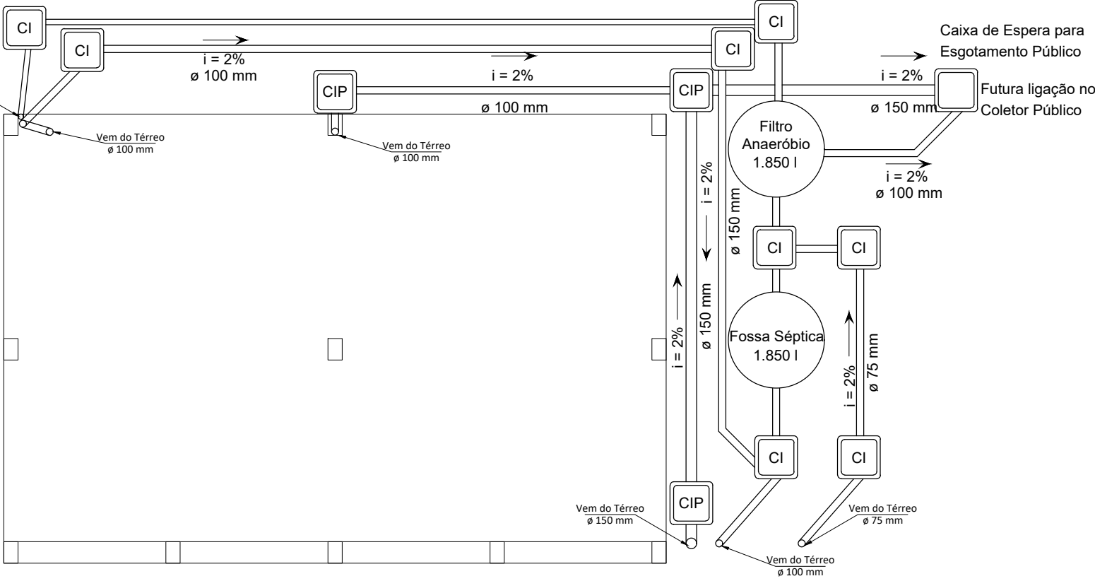
PLANTA BAIXA - SUB-SOLO (SANITÁRIO) ESC.: 1/75
