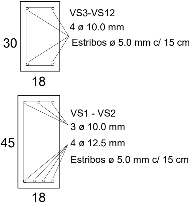
DETALHAMENTO VS - TÉRREO
