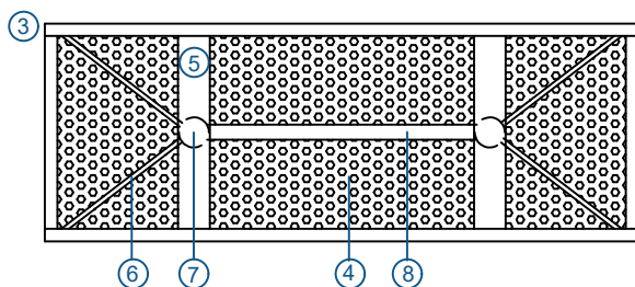
CORTE A-A (FUNDO DA LIXEIRA)
