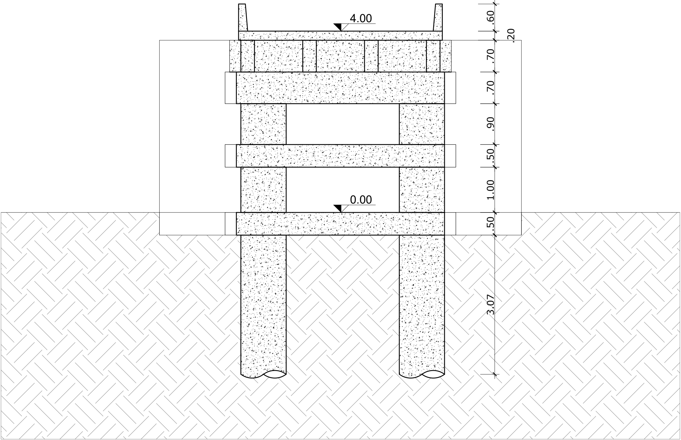
CORTE TRANSVERSAL Esc.:1/50
