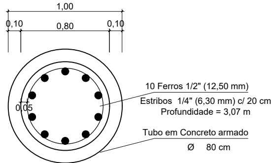
ESTACA DETALHAMENTO FERRAGEM
