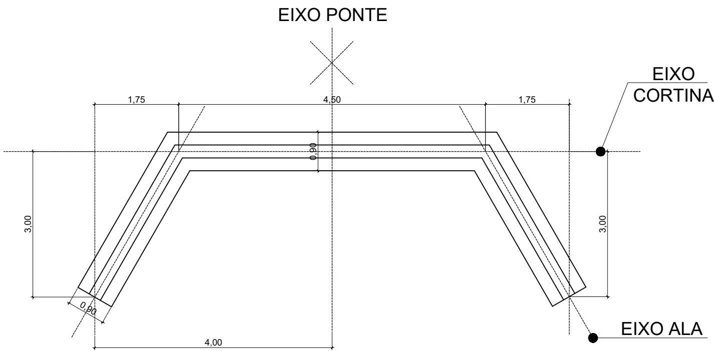
PLANTA MARCAÇÃO VIGA FUNDAÇÃO/CORTINA
