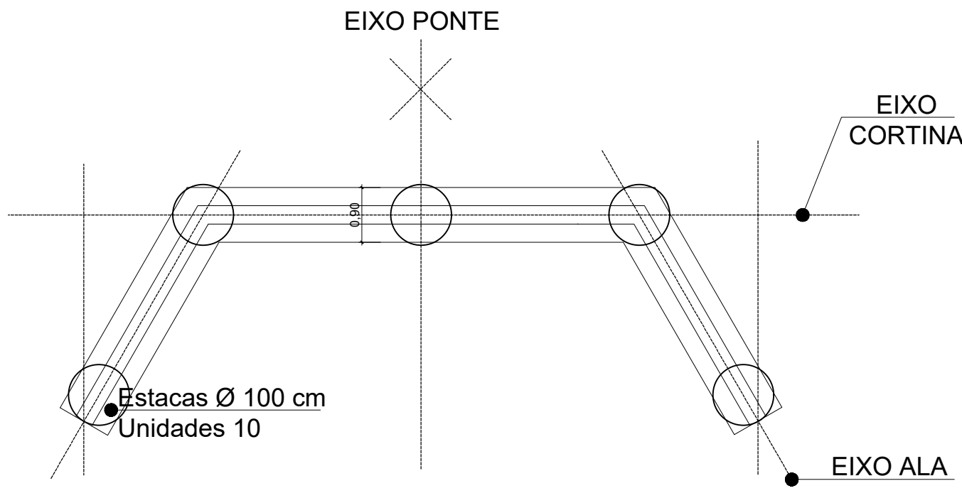
PLANTA LOCAÇÃO ESTACAS
