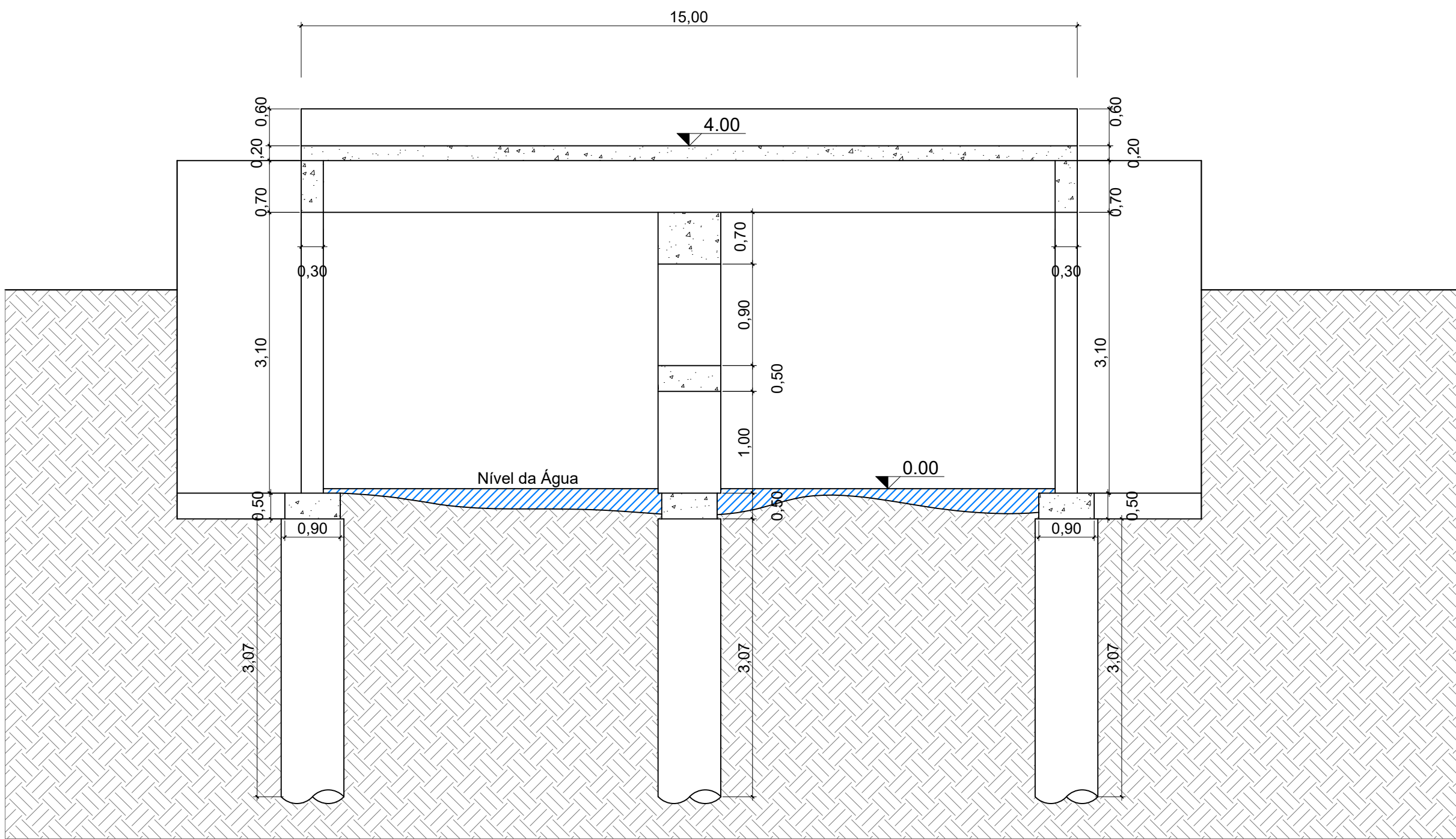
CORTE LONGITUDINAL
