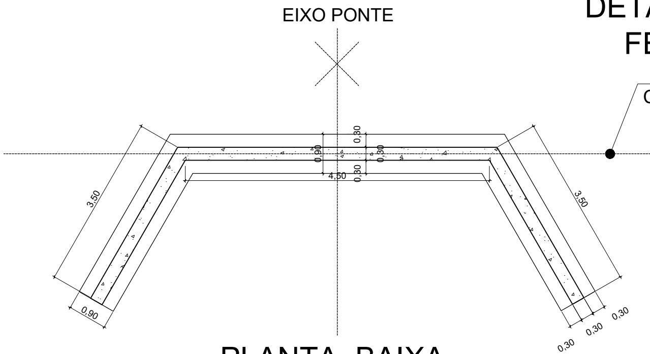
PLANTA BAIXA VIGA FUNDAÇÃO /CORTINA
