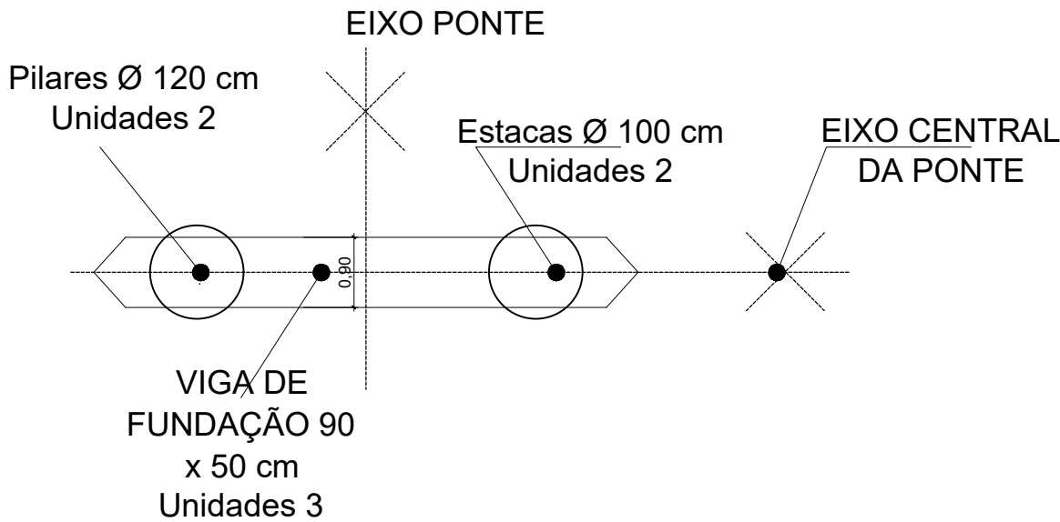
PLANTA LOCAÇÃO ESTACAS CENTRO DA PONTE
