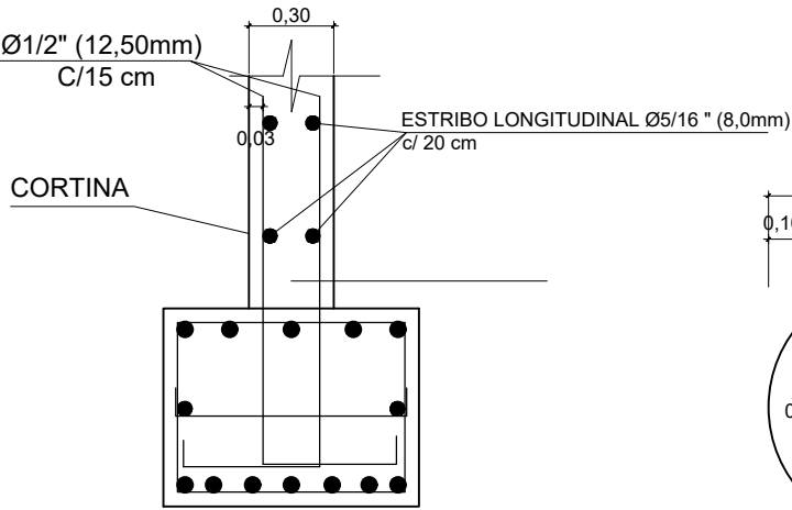
CORTINA DETALHAMENTO FERRAGEM
