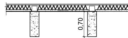
DETALHE ENGASTE TRELIÇAS
