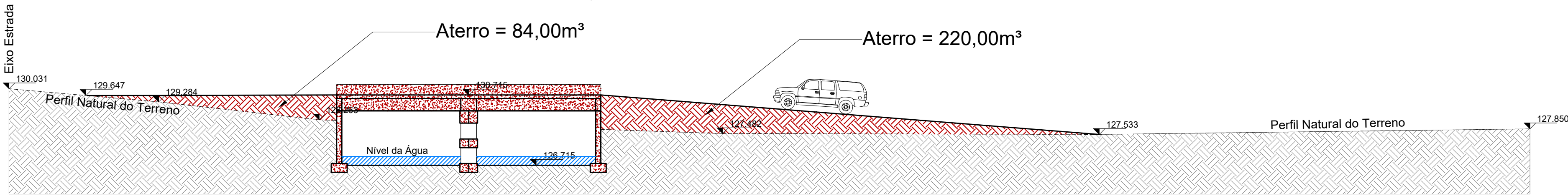
CORTE LONGITUDINAL - ATERRO S / ESC.
