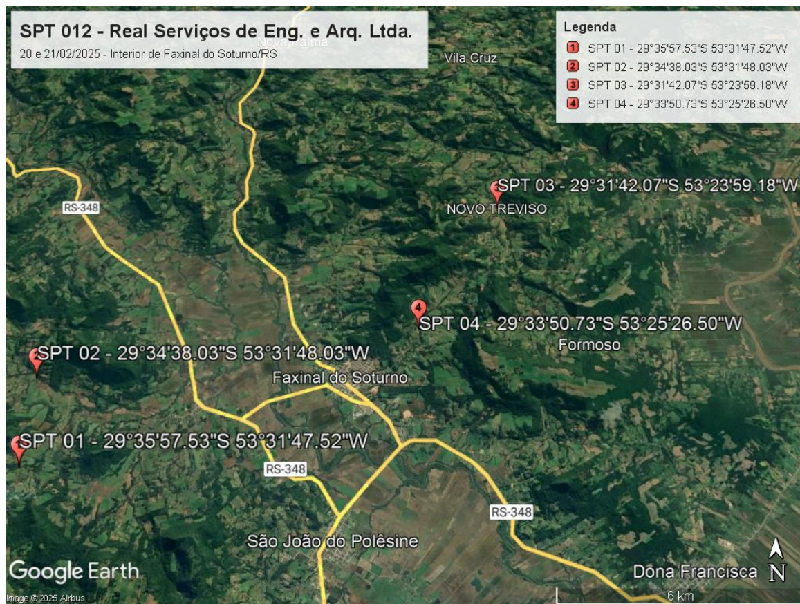
Figura 2 – Localização dos furos de sondagem SPT.
