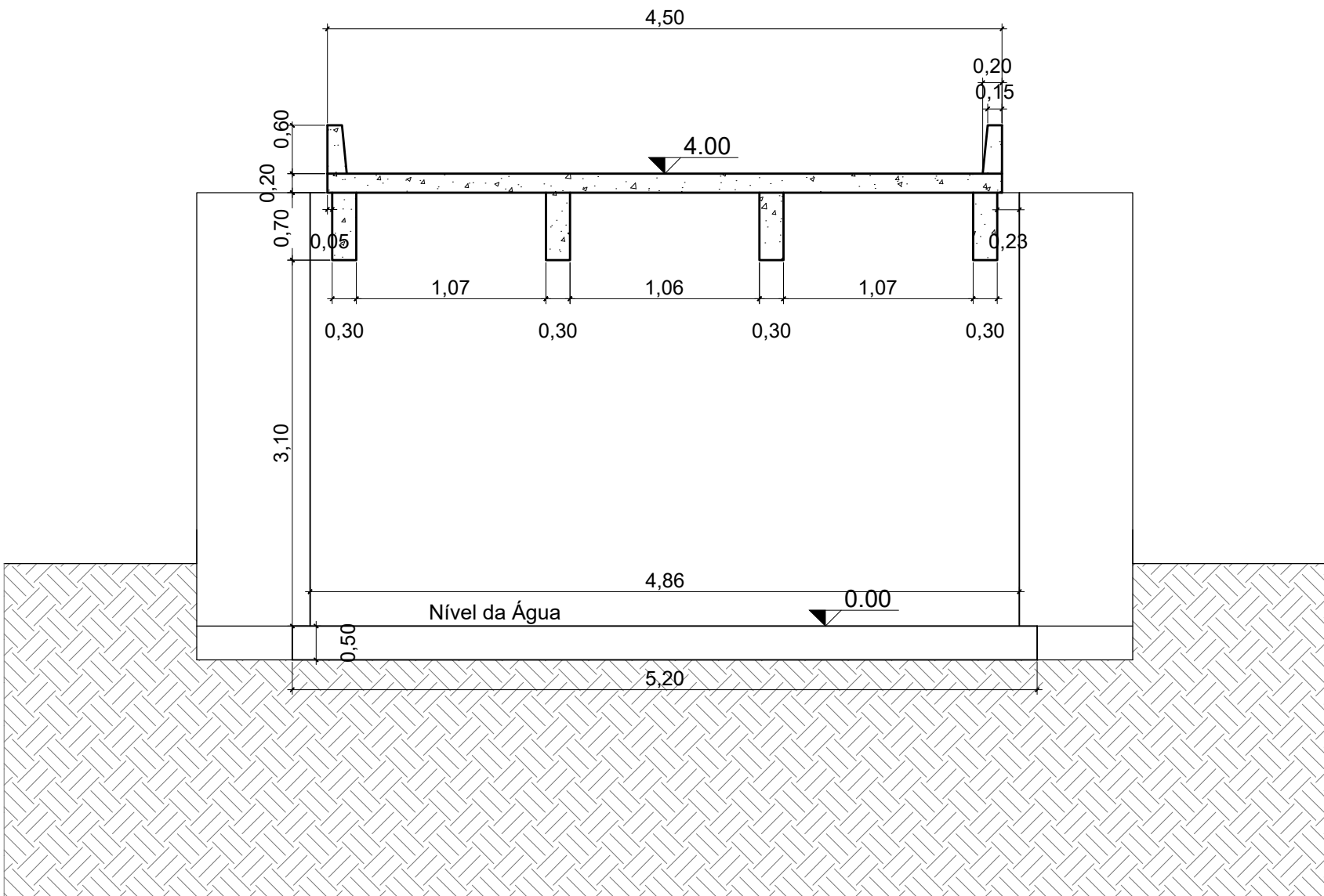
CORTE TRANSVERSAL
