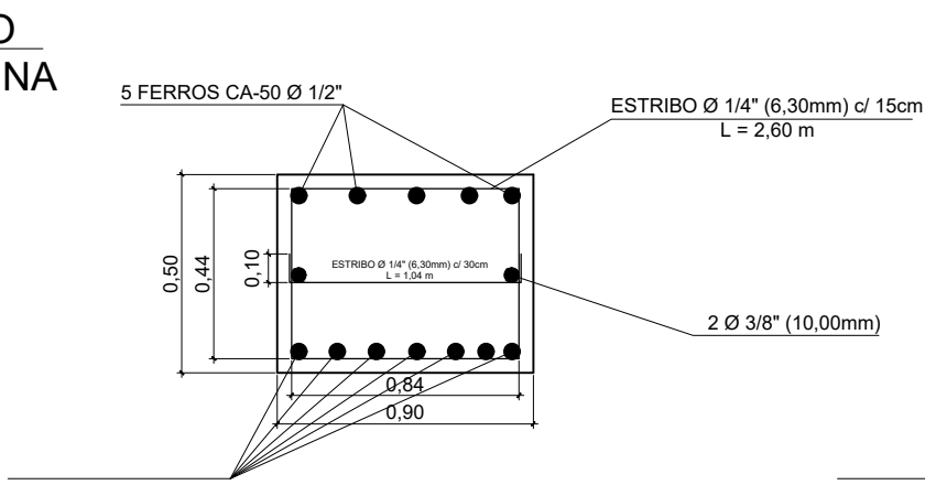
VIGA DE FUNDAÇÃO DETALHAMENTO FERRAGEM
