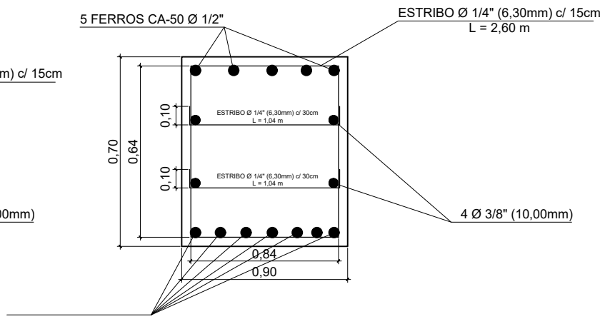
VIGA DE APOIO DAS LONGARINAS DETALHAMENTO FERRAGEM
