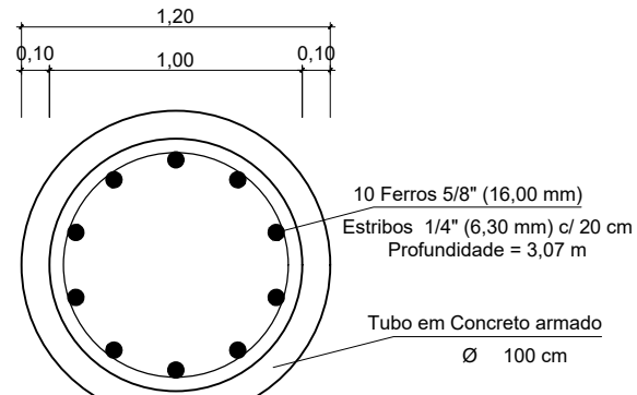
PILAR DETALHAMENTO FERRAGEM
