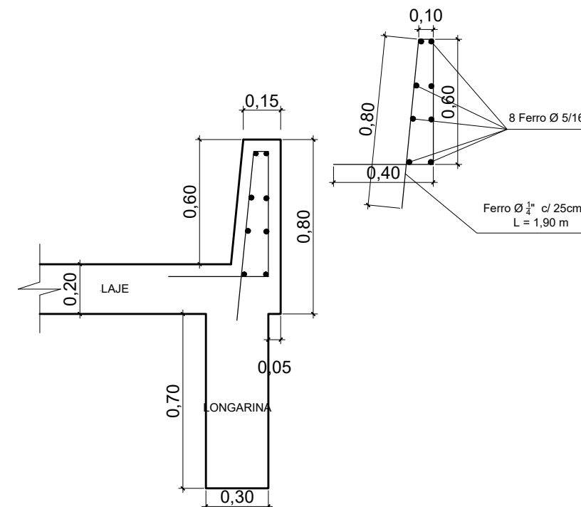
DETALHE FERRAGEM GUARDA CORPO
