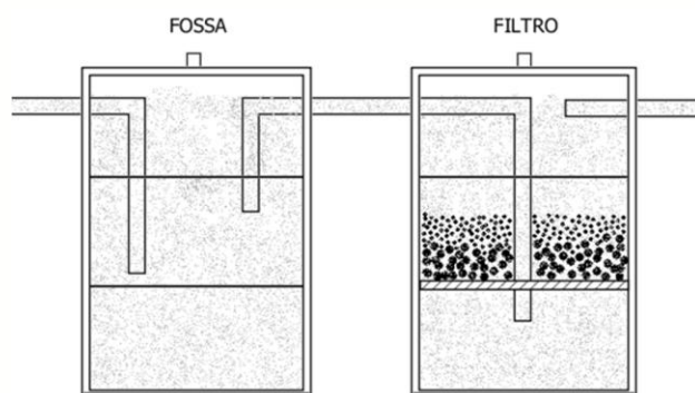
Figura 1 – Conjunto de tanque séptico e filtro anaeróbio
