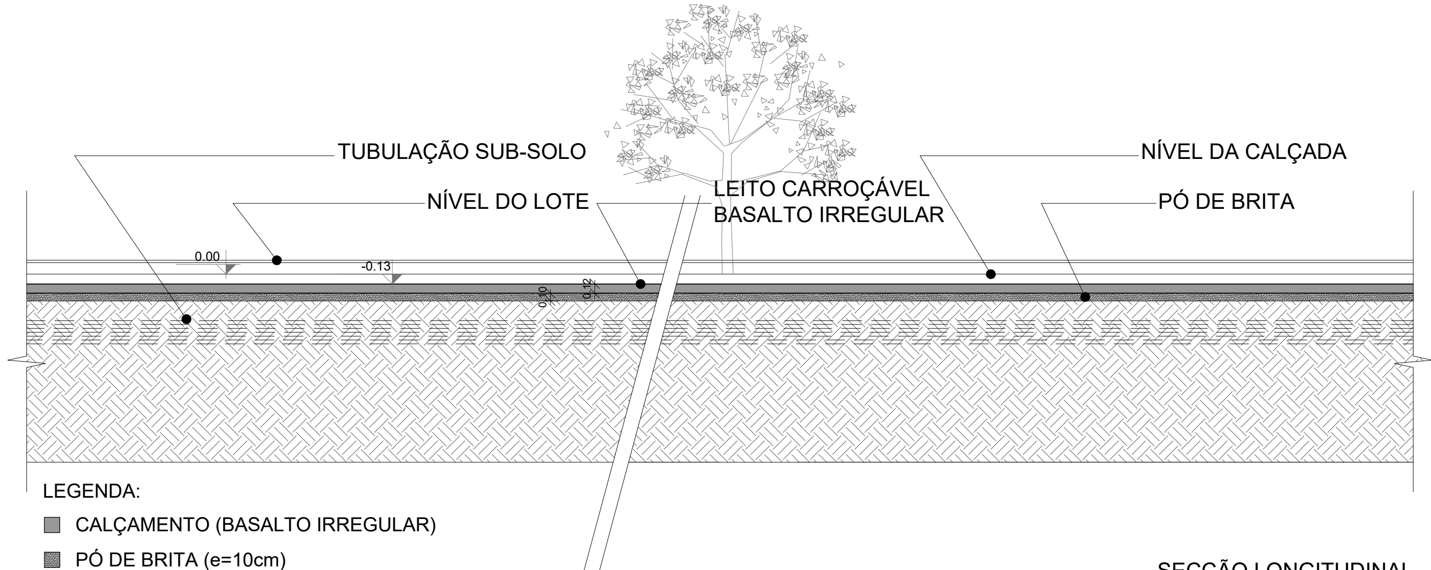
SECÇÃO LONGITUDINAL ESC.: 1/50
